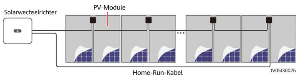
Abbildung 2-5 Verbotenes Kabelverlegung
