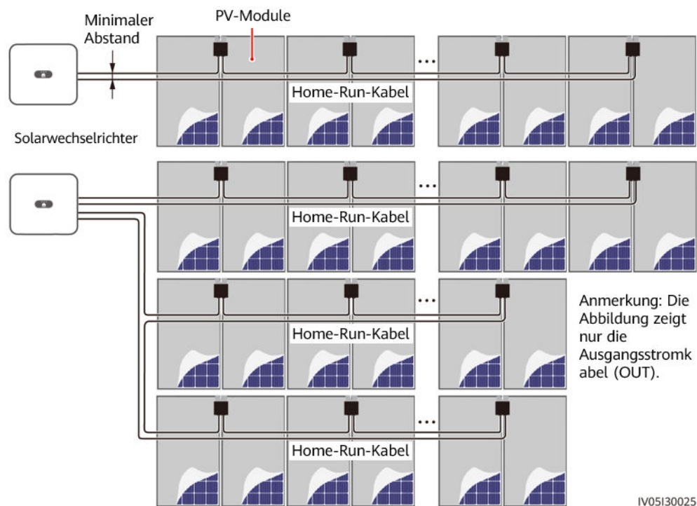
Abbildung 2-4 Erforderliches Kabelverlegung
