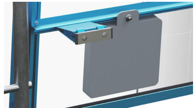
Rückansicht mit montiertem Mikro-Wechselrichter und Lift Adapter
