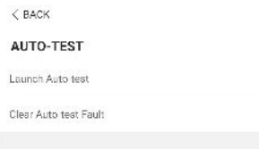
Abbildung 7-21 Automatischer Test
