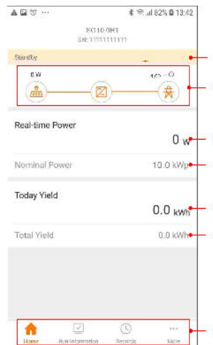
Abbildung 7-5 Startseite
