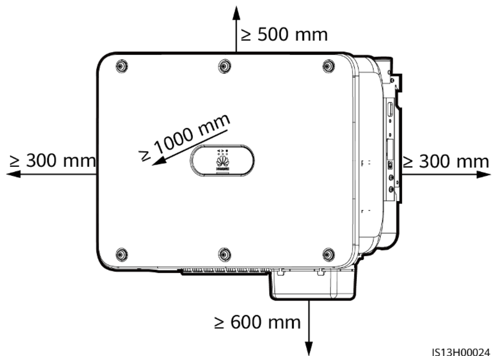
Abbildung 4-2 Montageabstände
