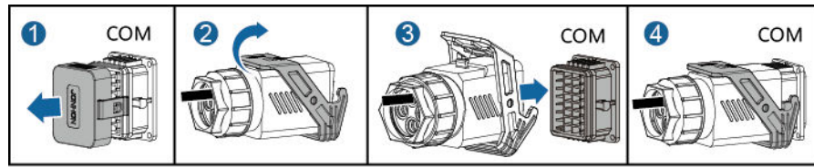
Abbildung 5-33 Sichern des Signalkabelanschlusses
