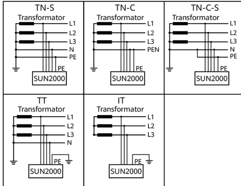
Abbildung 2-3 Stromnetze
