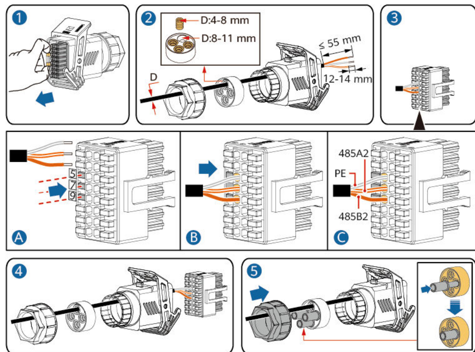
Abbildung 5-25 Kabelmontage
