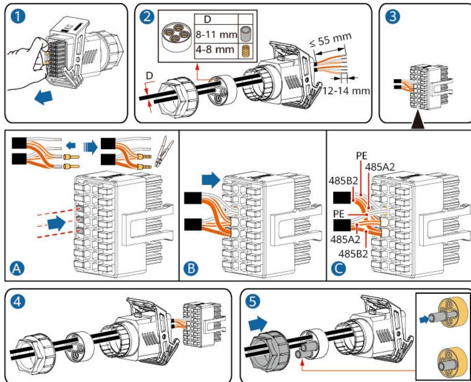
Abbildung 5-27 Kabelmontage
